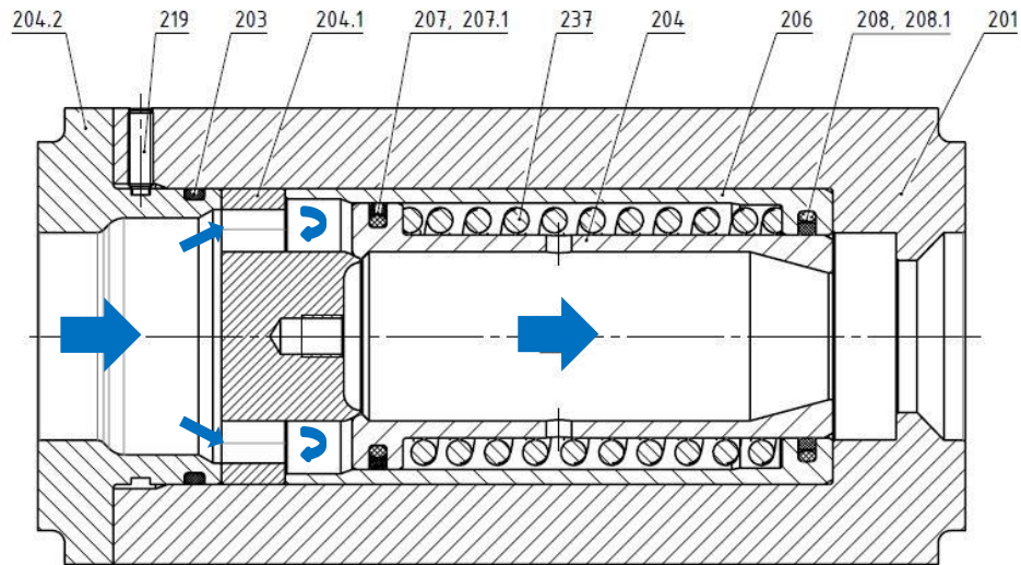
Figure 3 Robinetterie BPV (exécution Z) en état fermé
