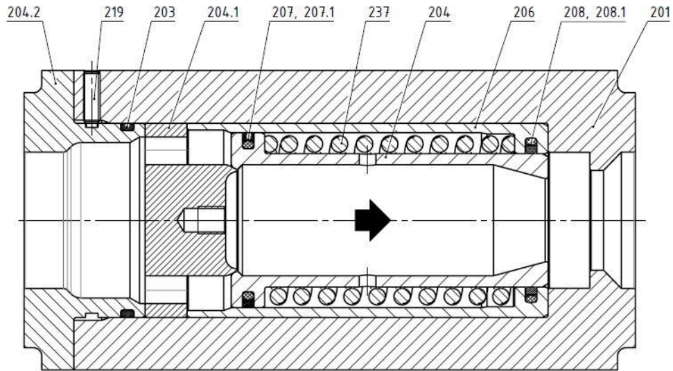
Figure 1 Plan en coupe du régulateur de pression en aval BPV (exécution Z)
