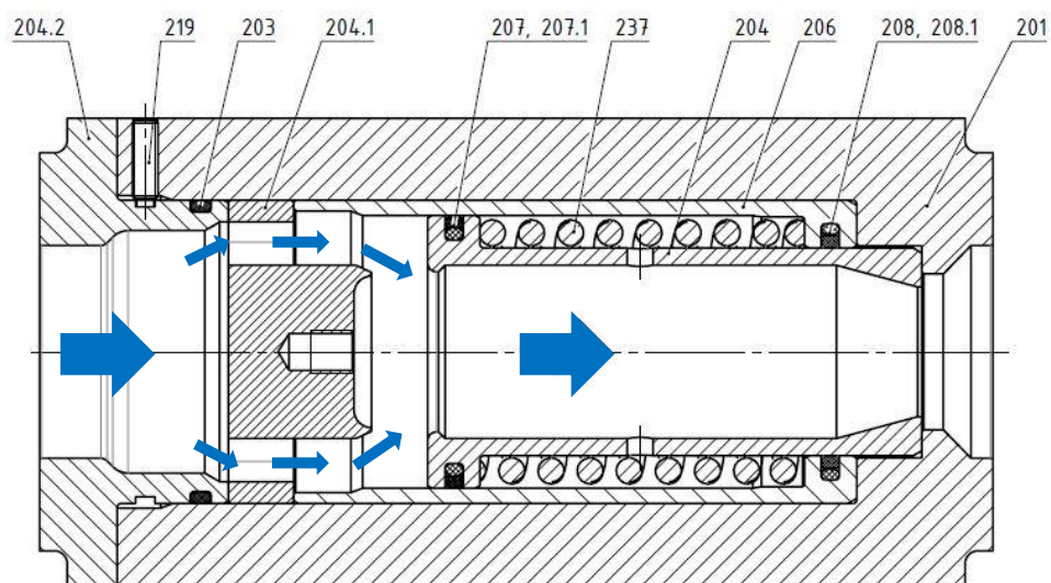
Figure 4 Robinetterie BPV (exécution Z) en état ouvert
