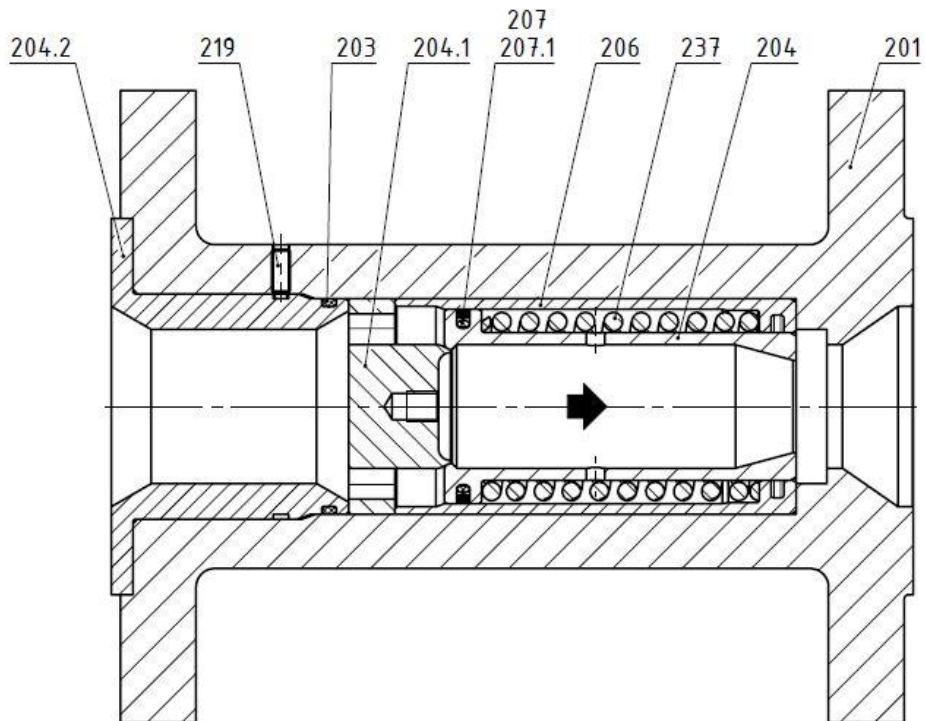
Figure 2 Plan en coupe du régulateur de pression en aval BPV (exécution K)
