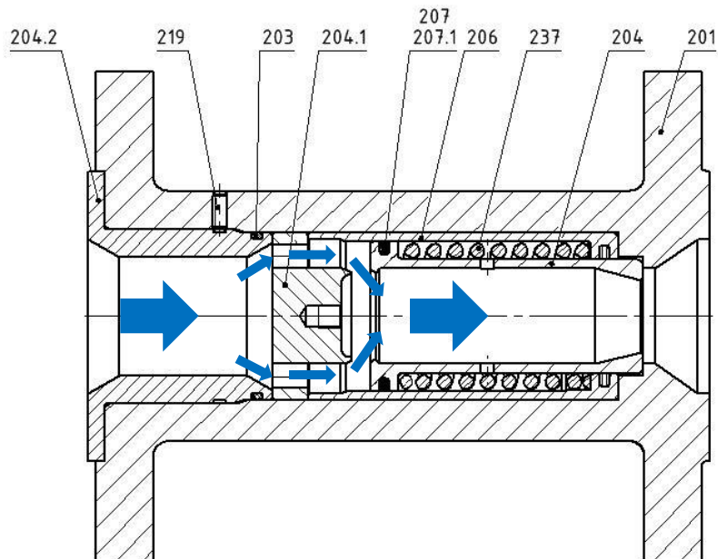
Figure 6 Robinetterie BPV (exécution K) en état ouvert
