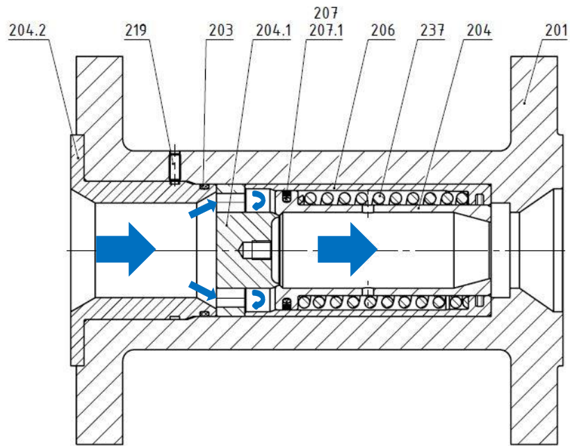
Figure 5 Robinetterie BPV (exécution K) en état fermé
