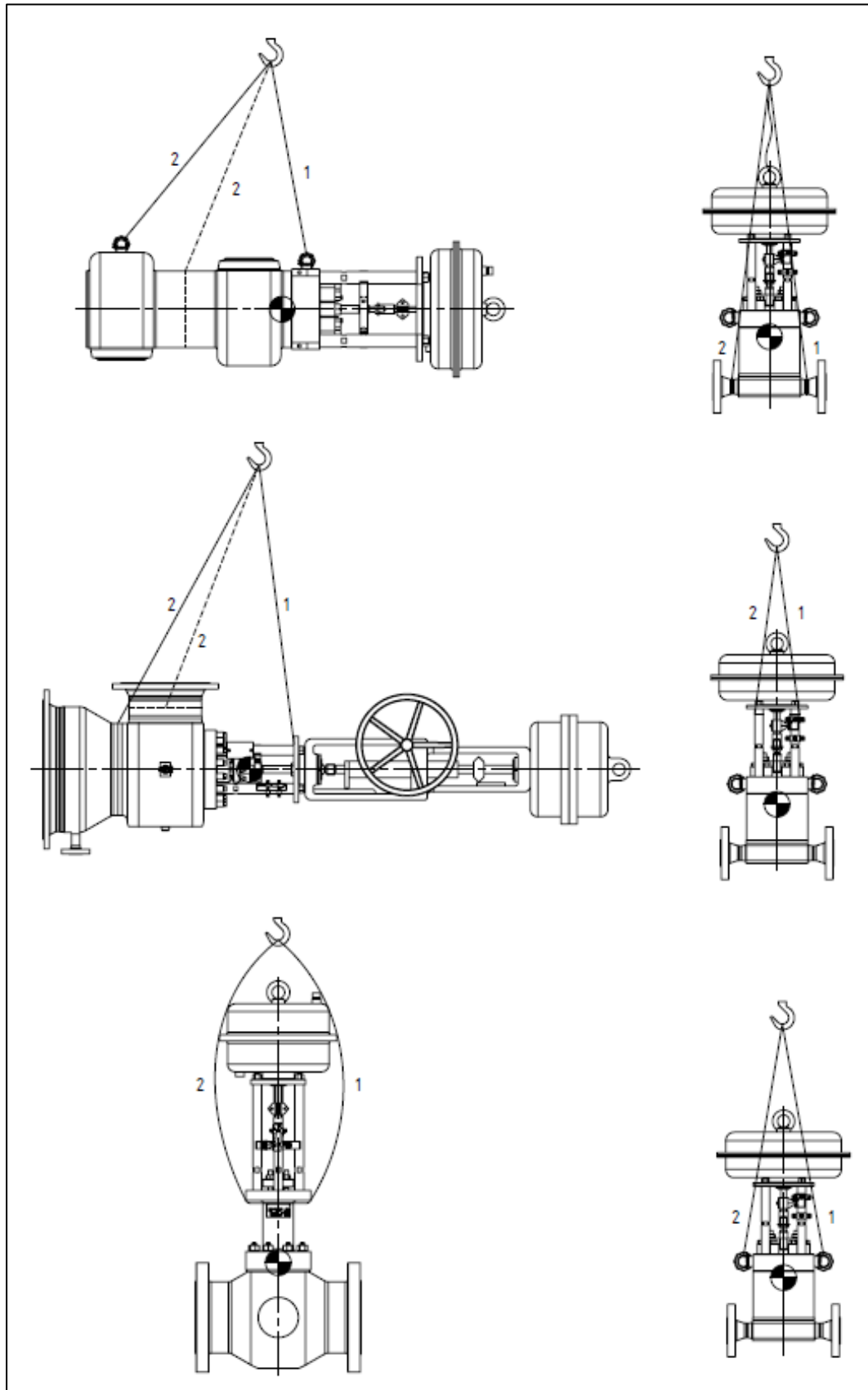
Figura 1 Muestra un ejemplo de las opciones de manipulación durante la instalación de la válvula. Las líneas discontinuas indican las opciones de sujeción alternativas.
