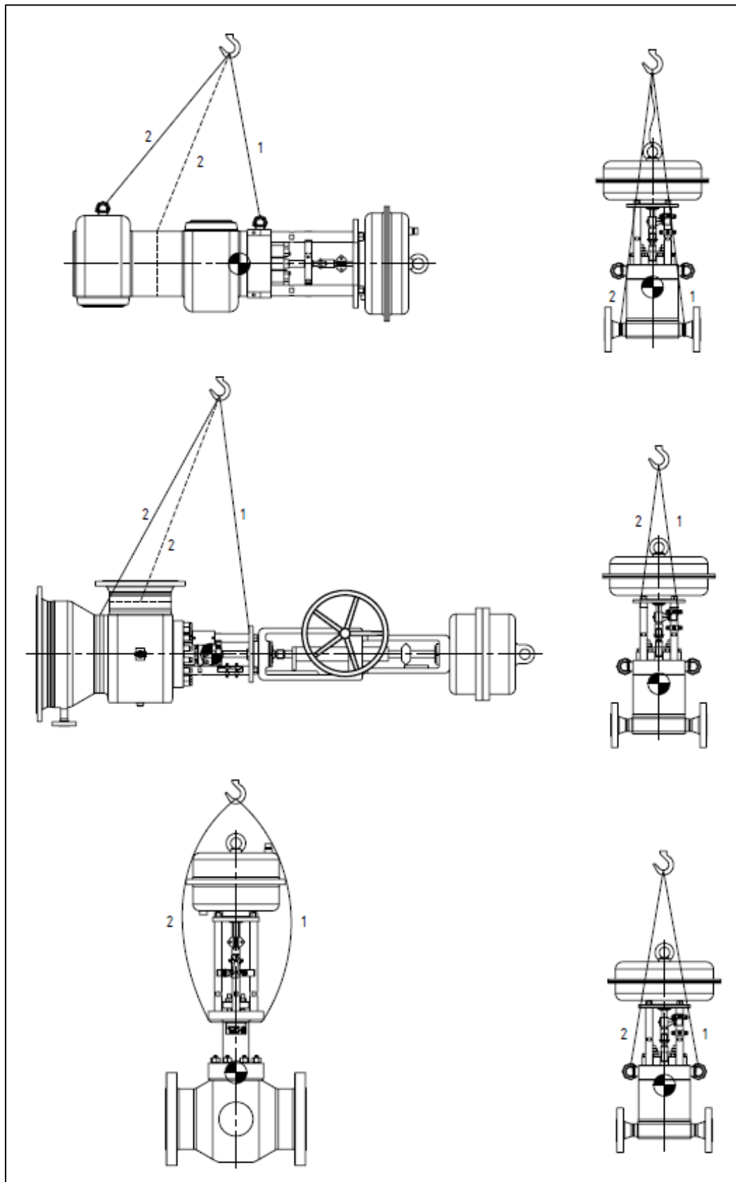
Figure 1 Exemple de représentation des possibilités de manipulation lors du montage de la robinetterie. Les lignes en pointillé indiquent les autres possibilités de fixation.
