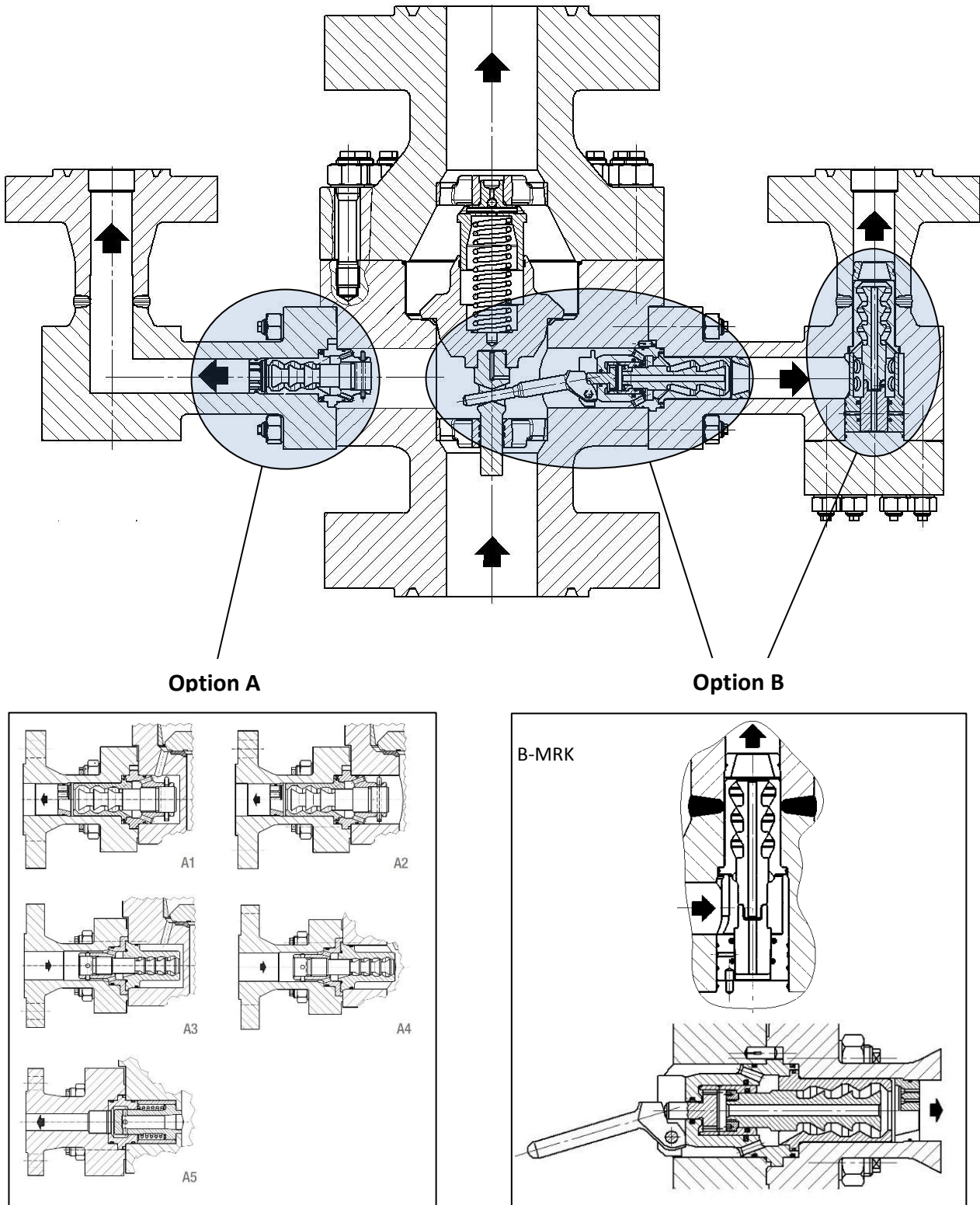
Abbildung 7 Armatur Typ MRK mit verschiedenen Anfahrstützen A1-A5 (links) und B-MRK (rechts)
