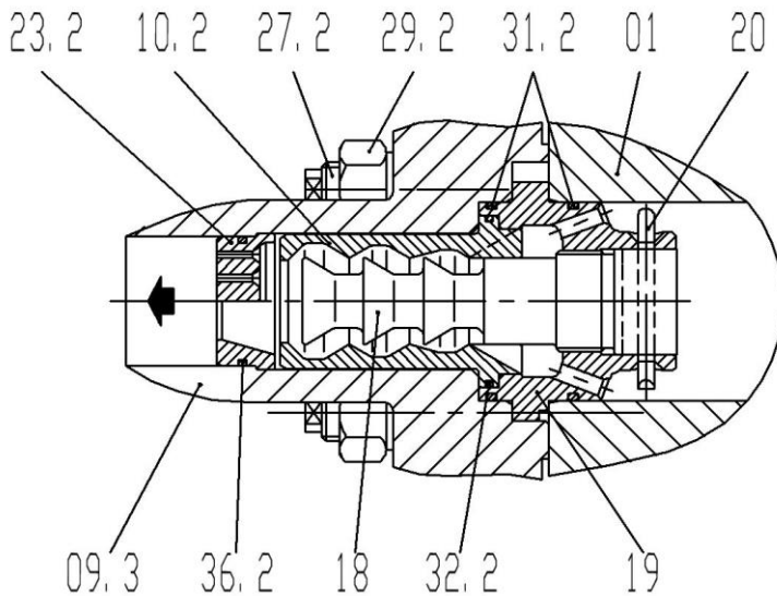
Abbildung 11 Manueller Anfahrstutzen mit Stückliste für Typ MRK
