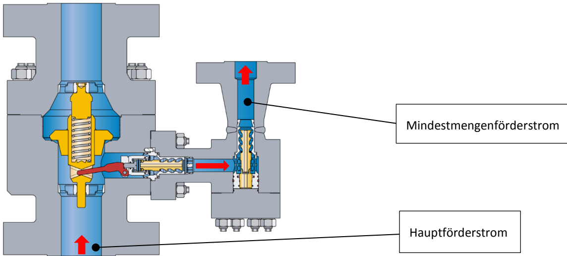
Abbildung 2 Armatur MRK mit geschlossenem Rückschlagkegel und geöffneten Freiläufen
