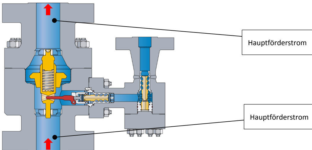
Abbildung 3 Armatur MRK mit geöffnetem Rückschlagkegel und sich gerade schließenden Freiläufen (Schaltpunkt)
