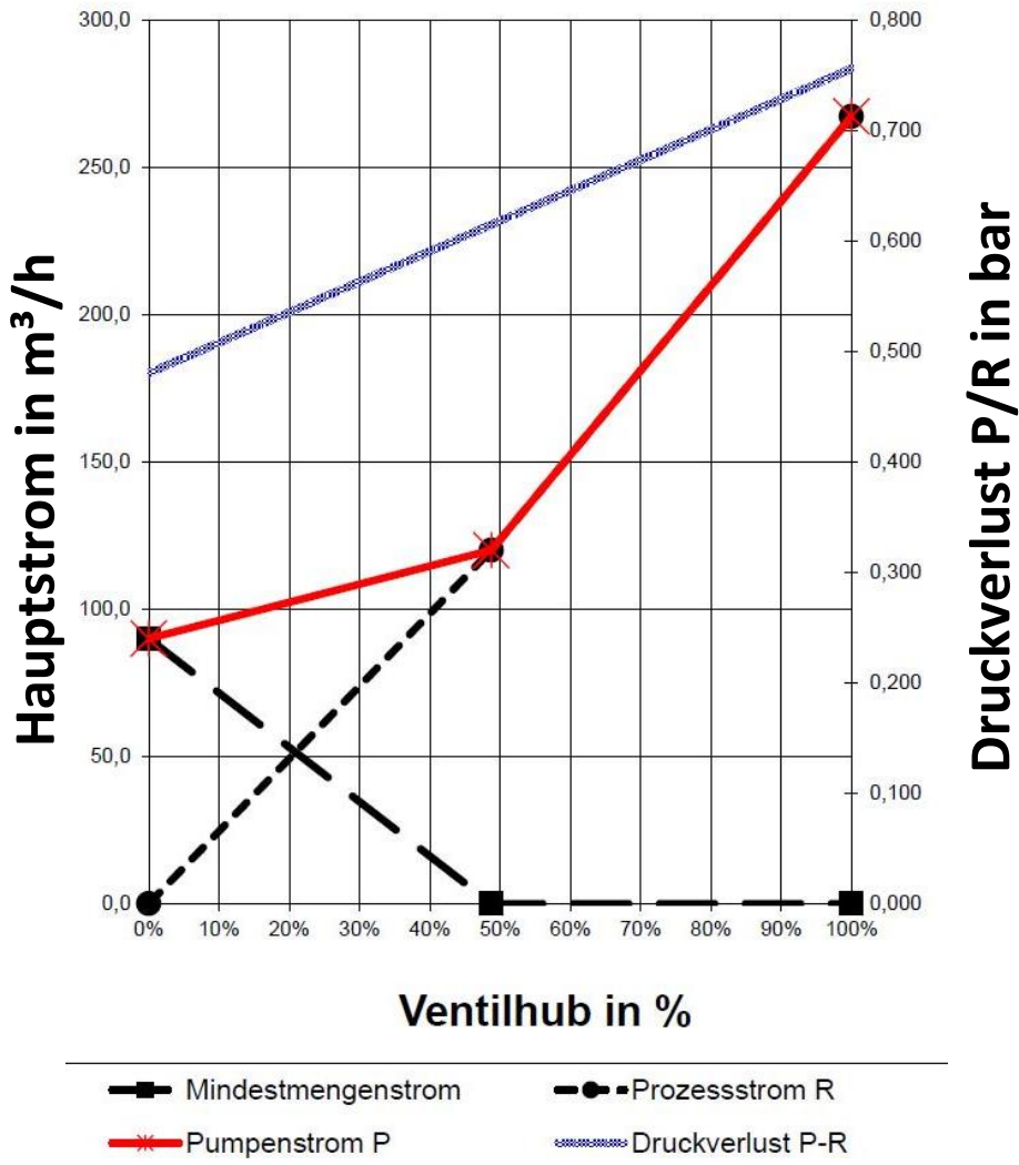
Abbildung 5 Kennlinie einer Mindestmengenarmatur des Typs MRK
