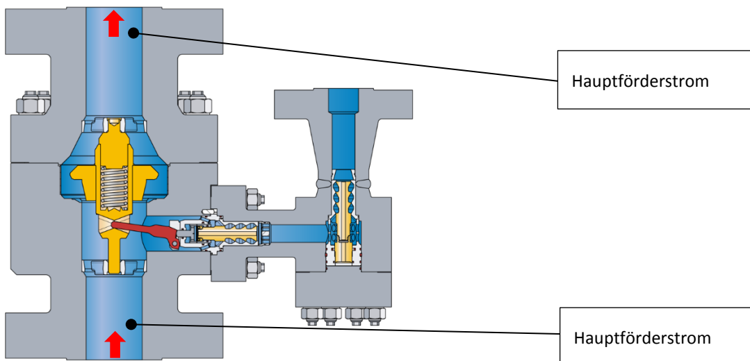
Abbildung 4 Armatur MRK mit geöffnetem Rückschlagkegel in maximaler Hubhöhe und geschlossenen Freiläufen
