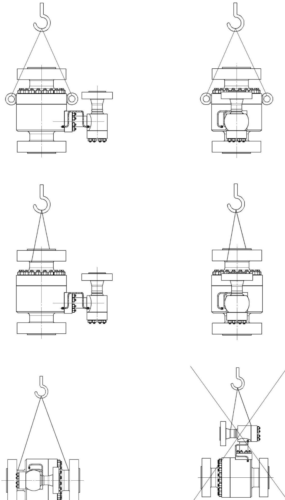
Abbildung 9 Beispielhafte Darstellung für die Handhabungsmöglichkeiten beim Einbau der Armatur
