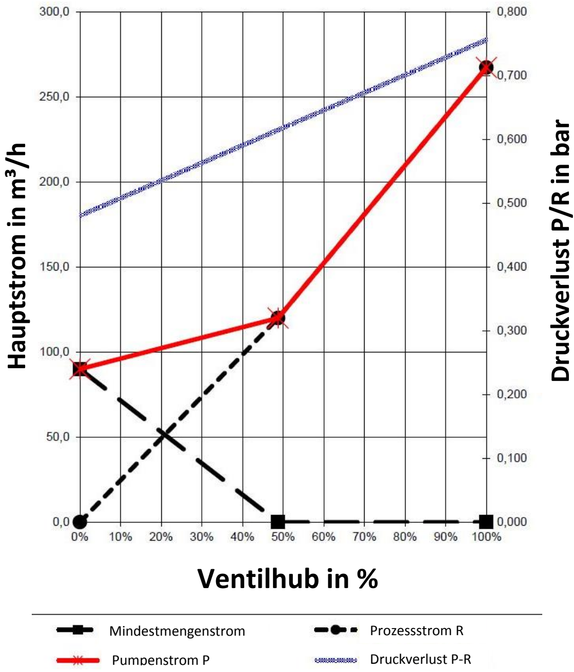
Abbildung 6 Kennlinie einer Mindestmengenarmatur des Typs SUL
