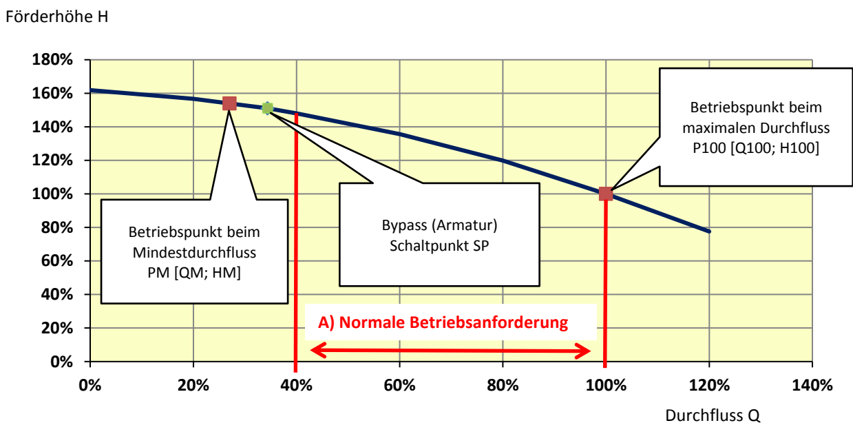
Abbildung 7 Normale Betriebsanforderung
