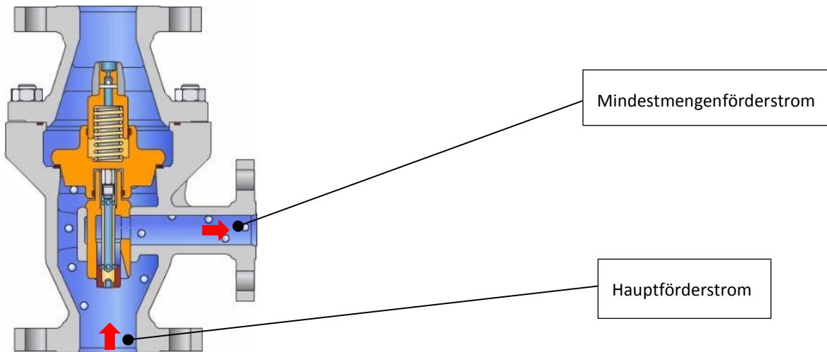
Abbildung 3 Armatur SUL mit geschlossenem Rückschlagkegel und geöffnetem Freilauf
