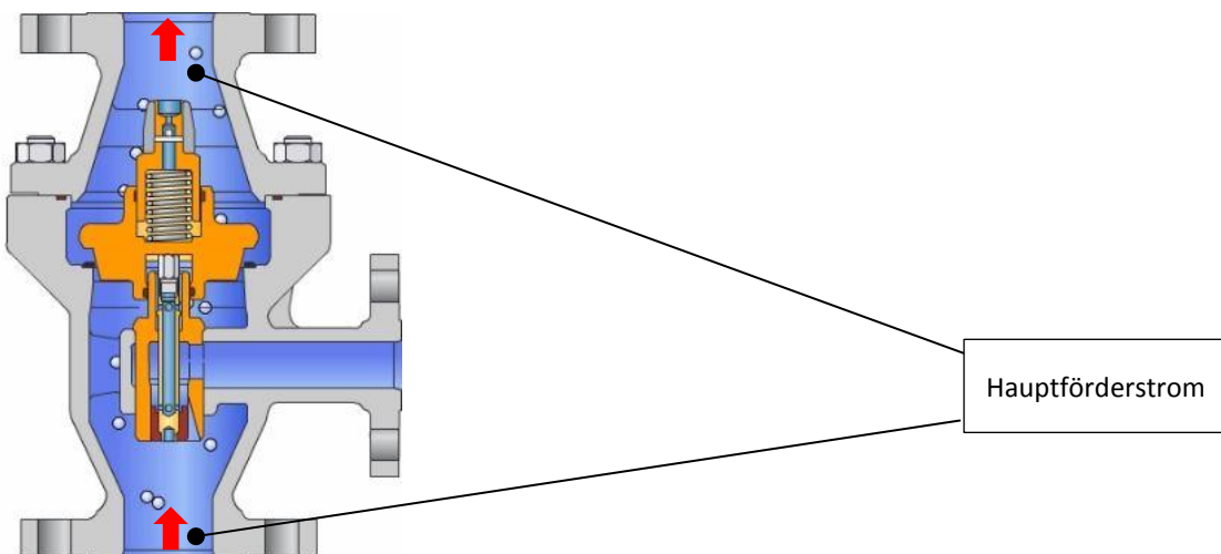
Abbildung 4 Armatur SUL mit geöffnetem Rückschlagkegel und sich gerade schließendem Freilauf (Schaltpunkt)
