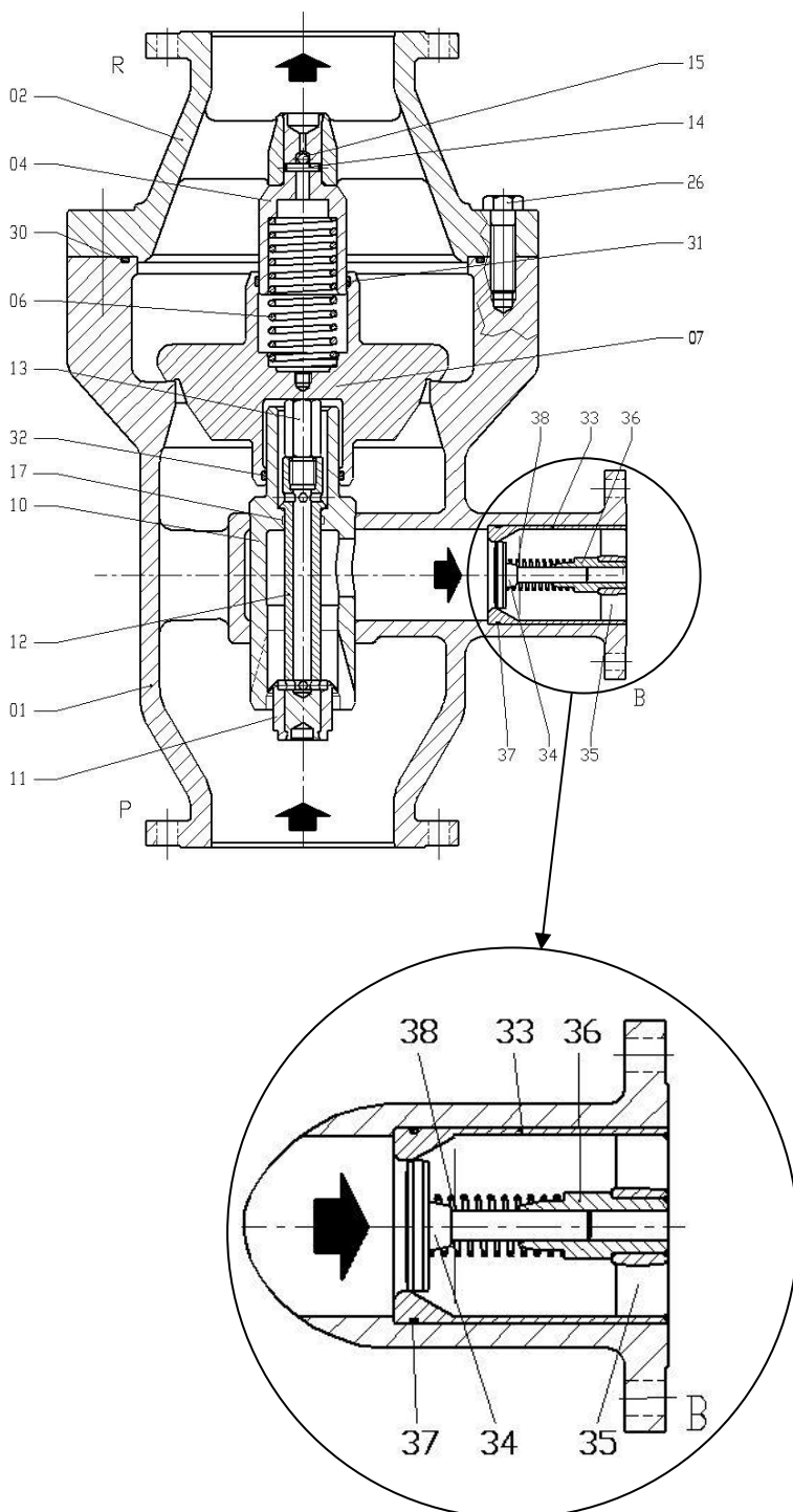
Abbildung 2 Schnittzeichnung und Stückliste der Armatur Typ SUL mit Rückschlagfunktion (Beispiel)
