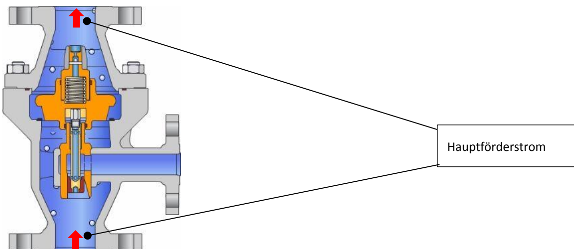
Abbildung 5 Armatur SUL mit geöffnetem Rückschlagkegel in maximaler Hubhöhe und geschlossenem Freilauf
