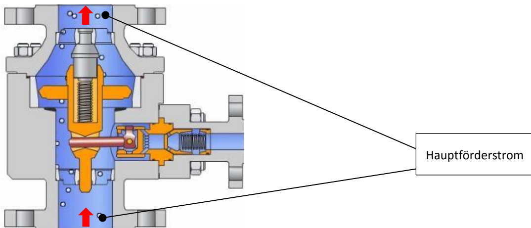
Abbildung 4 Armatur TDL mit geöffnetem Rückschlagkegel und sich gerade schließendem Freilauf (Schaltpunkt)
