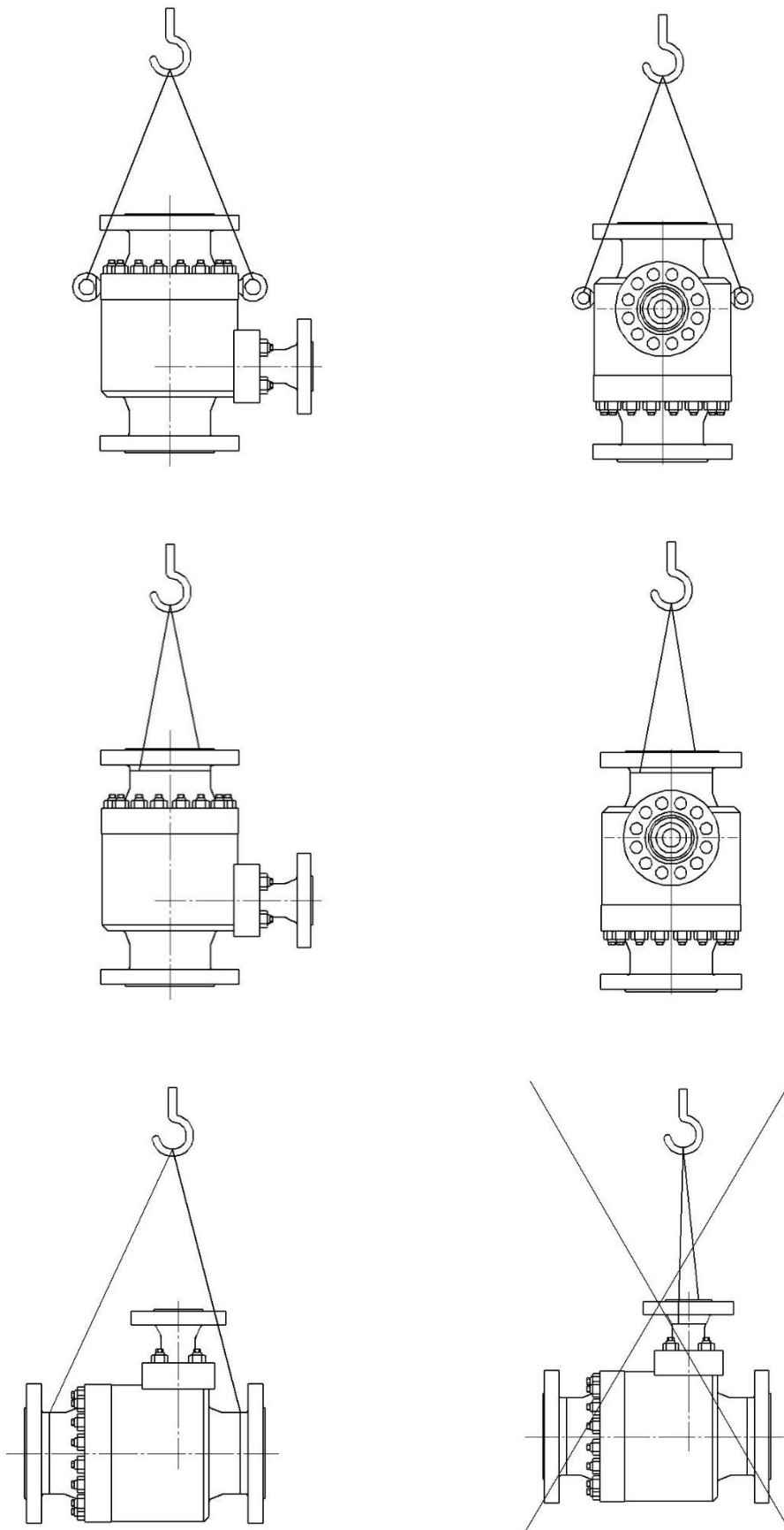
Abbildung 10 Beispielhafte Darstellung für die Handhabungsmöglichkeiten beim Einbau der Armatur
