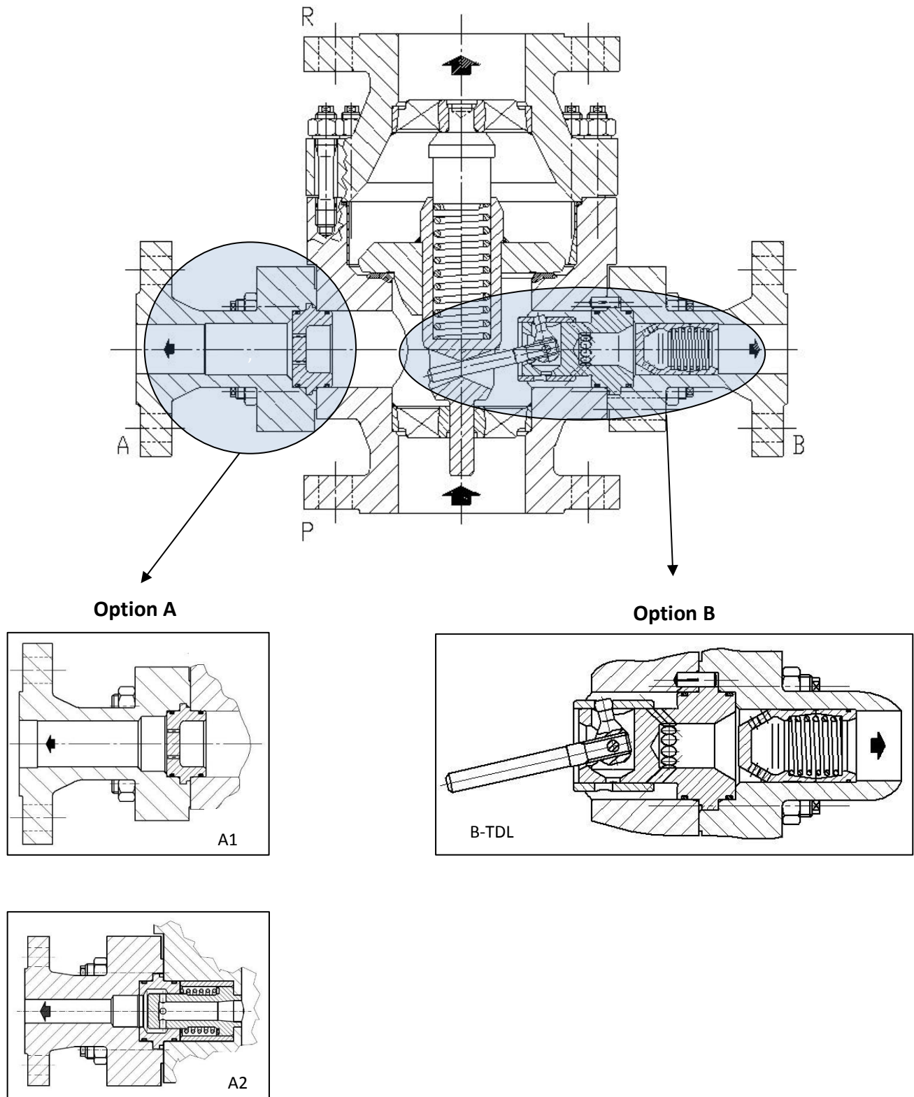
Abbildung 8 Armatur Typ TDL mit verschiedenen Anfahrstützen A1 u. A2 (links) und B-TDL (rechts)
