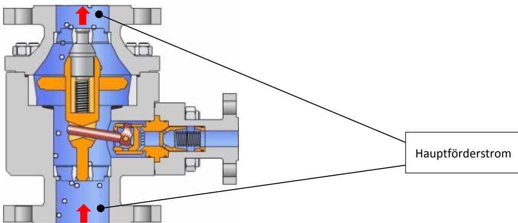
Abbildung 5 Armatur TDL mit geöffnetem Rückschlagkegel in maximaler Hubhöhe und geschlossenem Freilauf
