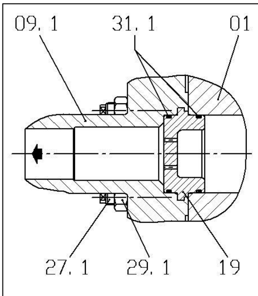
Abbildung 12 Manueller Anfahrstutzen Typ TDL mit Stückliste
