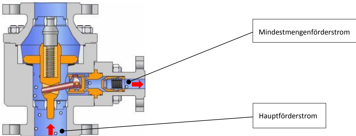
Abbildung 3 Armatur TDL mit geschlossenem Rückschlagkegel und geöffnetem Freilauf
